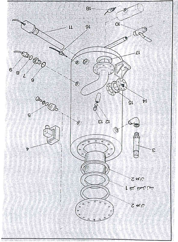
فانل قاصل الزيت و الهواء Oil & Air Separator
